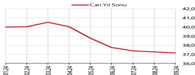
Grafik 9: Cari Yıl Sonu ABD Dolar Kuru Beklentisi ($/TL)
