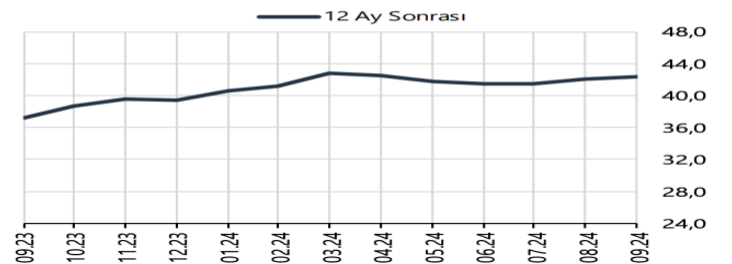
Grafik 10: 12 Ay Sonrası ABD Dolar Kuru Beklentisi ($/TL)
